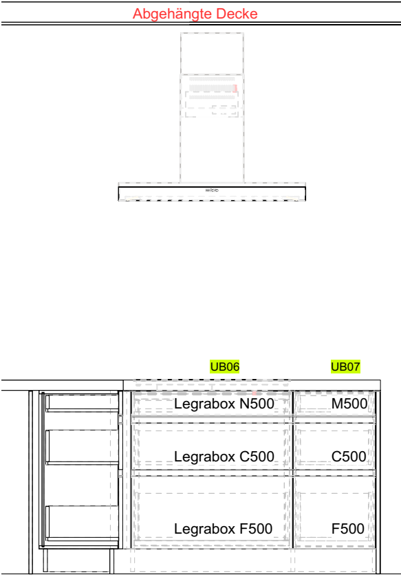
Ansicht E-E
