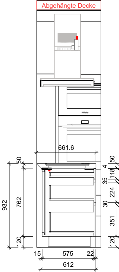
Abgehängte Decke
