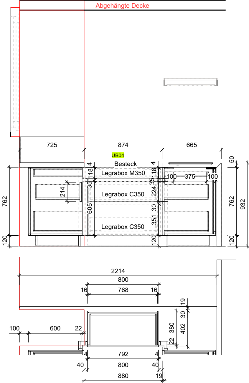
Ansicht D-D
